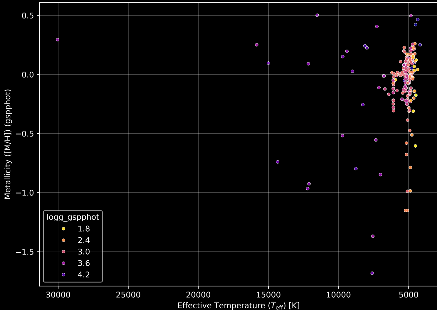
APOGEE DR17 Field: [143-04] Stellar Population Parameters (n= 204)
